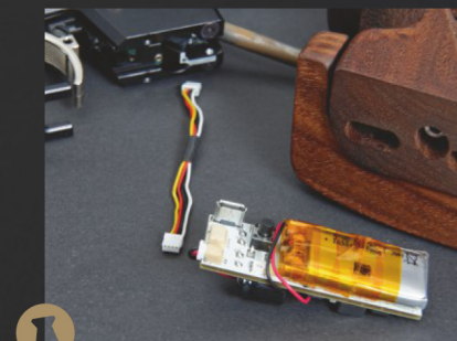
Kabel beim Elektronikmodul austauschbar (E) Exchangeable cable at the electronic module (E)
